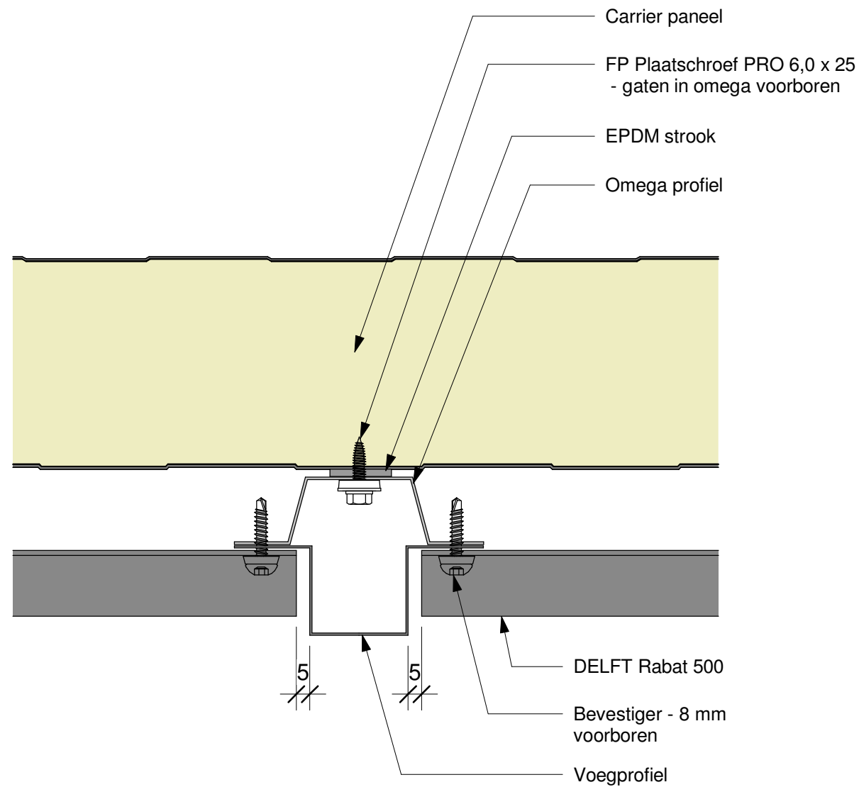
Detail - Stuiknaad met voegprofiel
